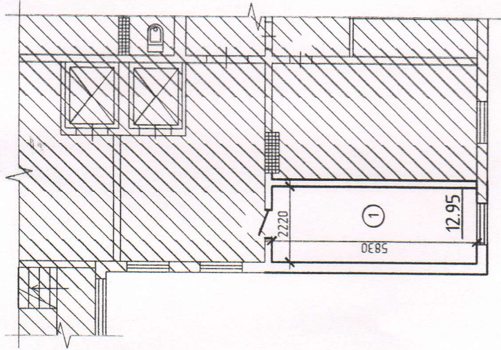
Обмірний план
